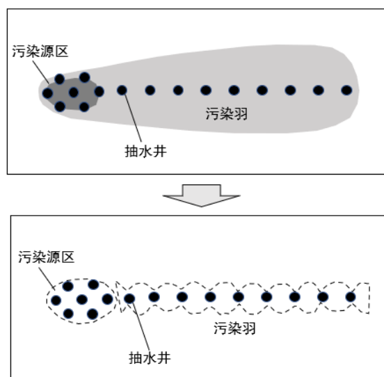
图4 污染羽修复策略抽水井布设示意图
