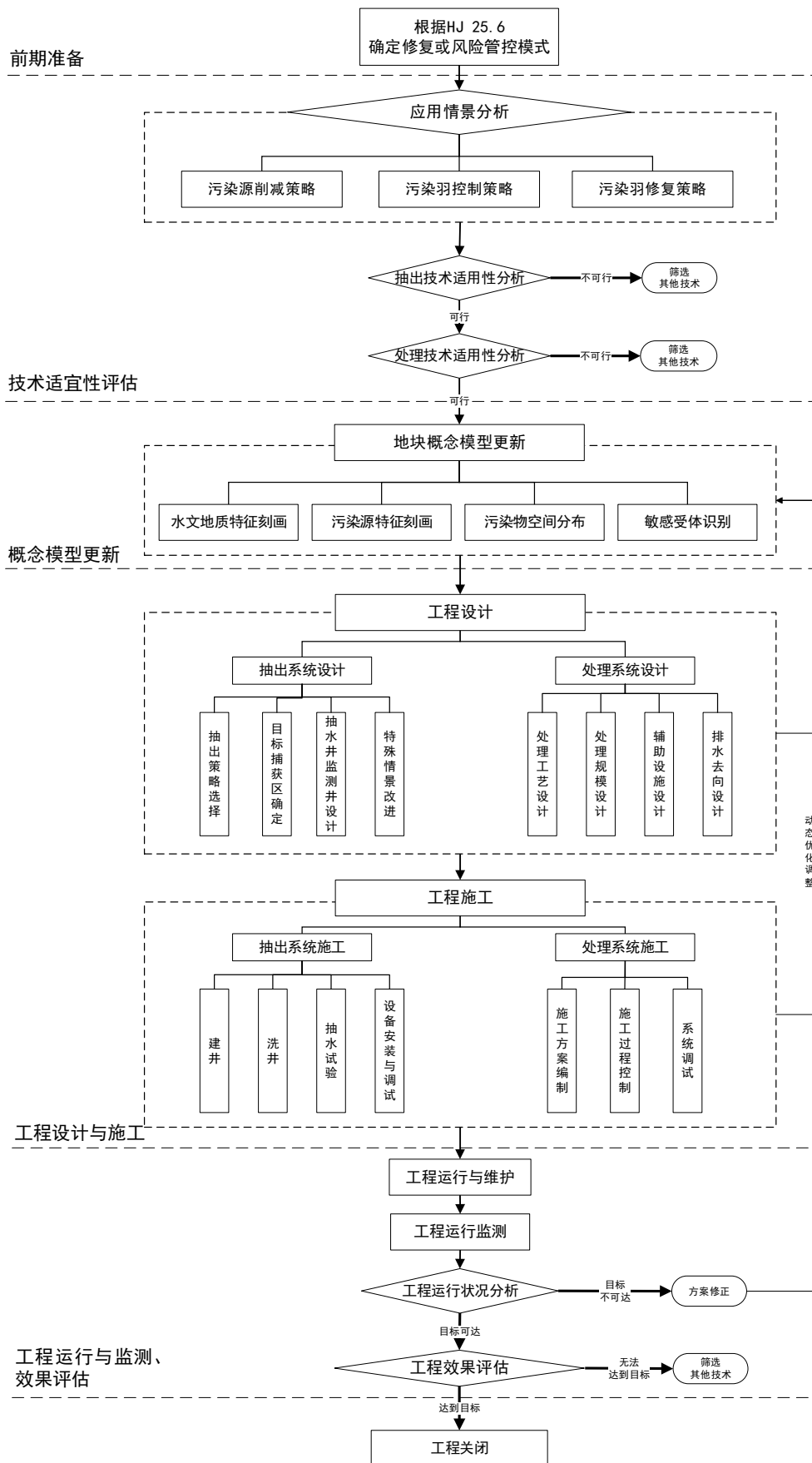
图 1 抽出一处理技术工作流程图
