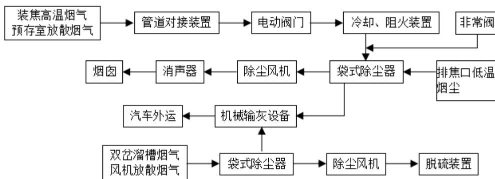
图 12 干熄焦除尘地面站工艺流程
