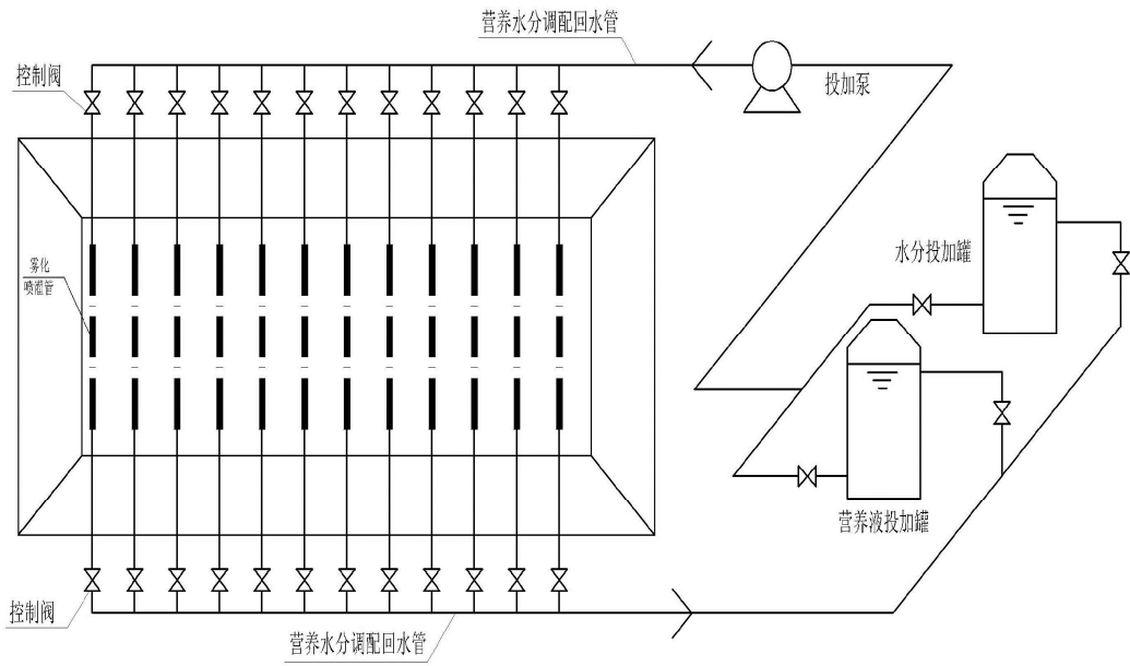
图 D. 3 营养及水分调配系统平面布置示意图
