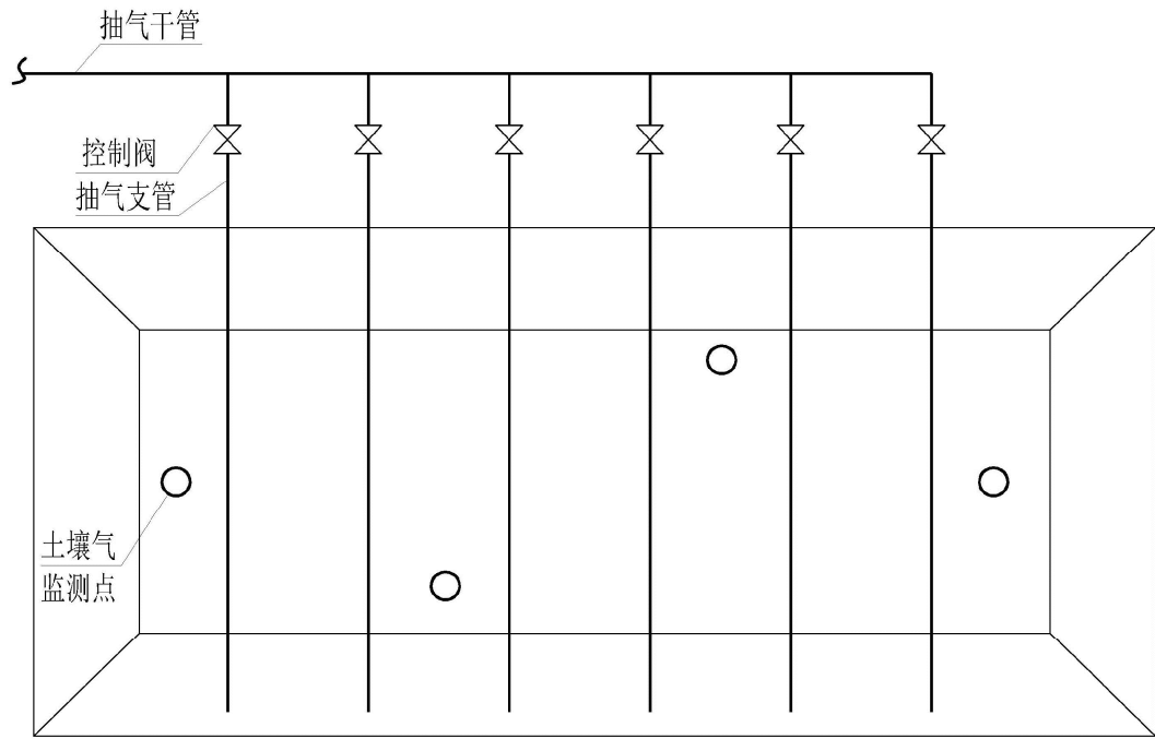
图 C.2 土壤气监测点平面布置示意图
