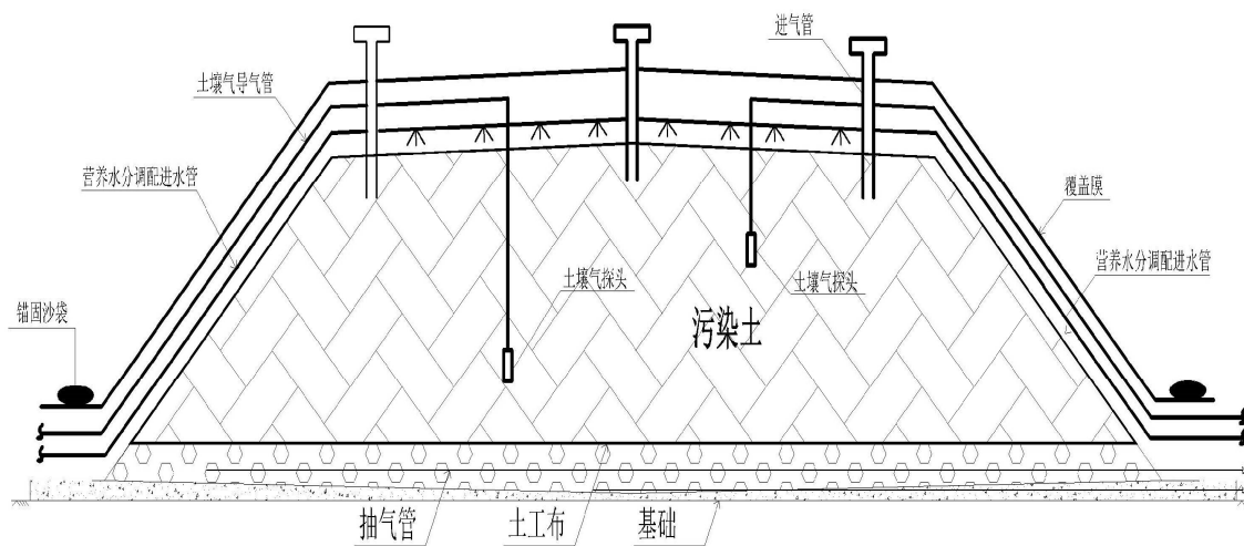
图 D. 1 系统剖面示意图
