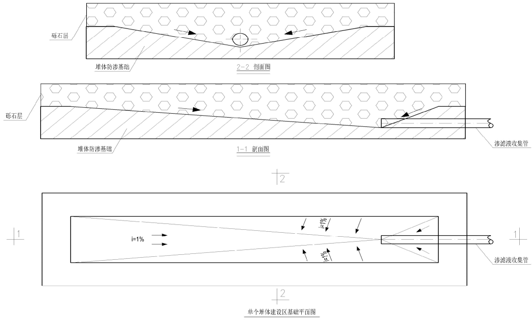
图 B.1 堆体底部防渗与渗滤液收集系统示意图
