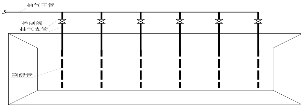
图 B.2 堆体底部抽气管平面布置示意图
