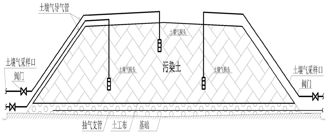
图 C.3 土壤气监测点垂向布置示意图
