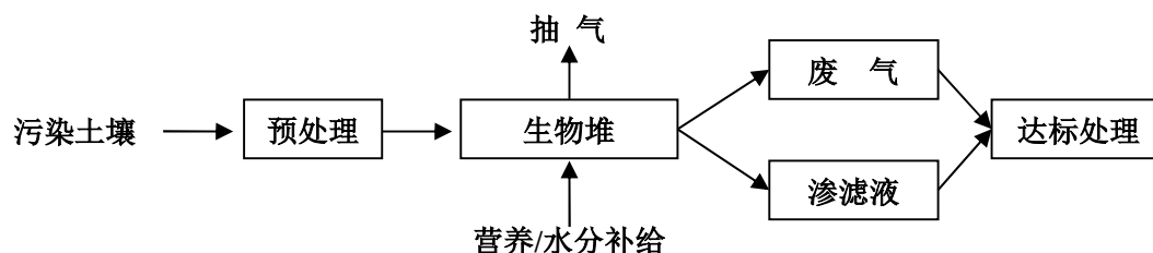
图 1 生物堆修复污染土壤的工艺流程
