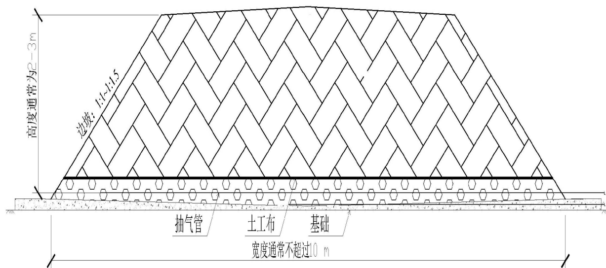
图 C. 1 堆体剖面示意图
