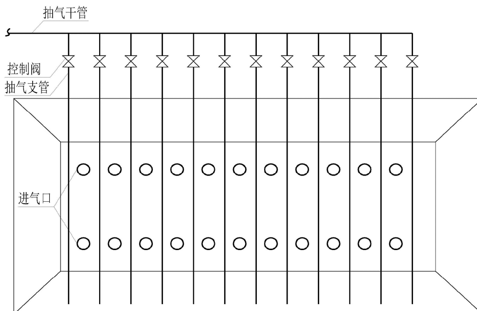
图 D. 2 进气管平面布置示意图
