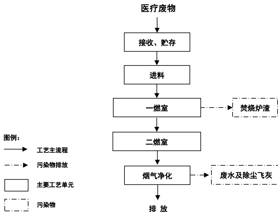
图 1 医疗废物集中焚烧处置一般工艺流程图
