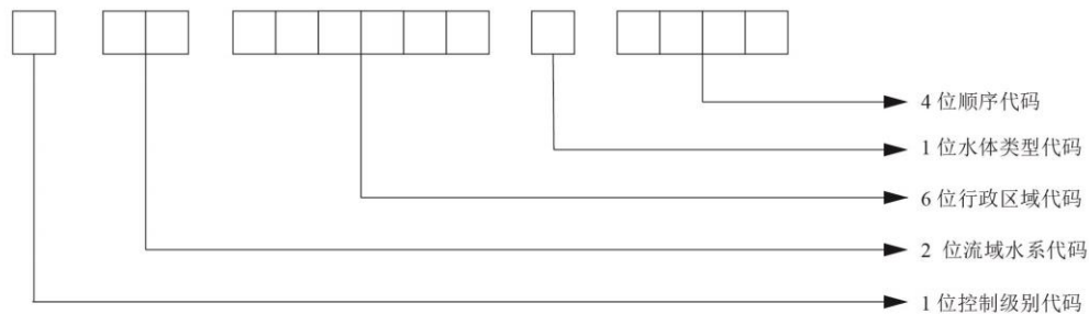
图 1 代码结构图
